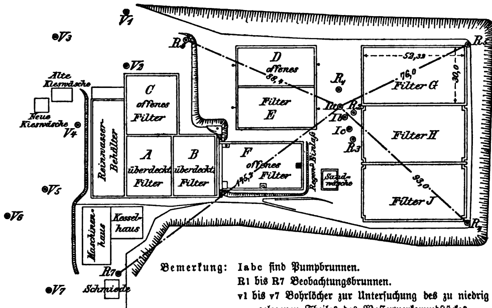
Lageplan von dem Wasserwerkgrundstück der Stadt Stettin in Pommerensdorf mit den ausgeführten Bohrlöchern.
