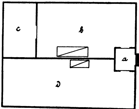
Fig. 5. Küchengebäude. a Vorraum. — b Küche. — c Speisesammer. — d Speisesaal.
