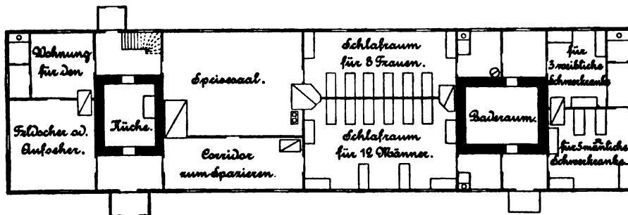
Fig. 7. Leprosorium in Ruda. Hauptgebäude.
