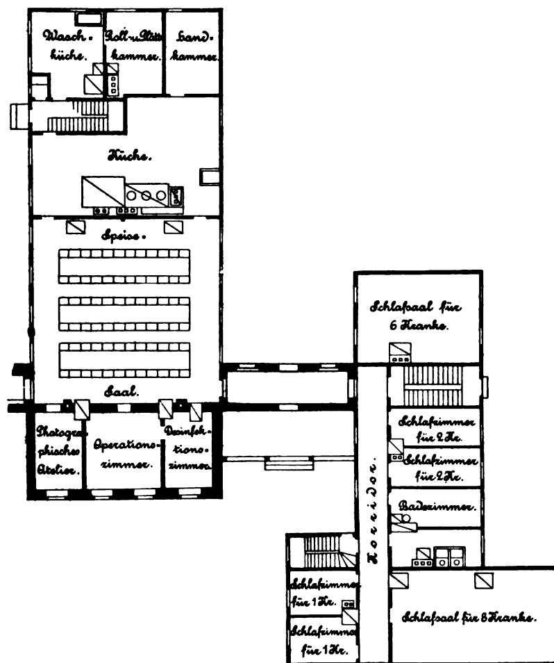
Fig. 13. Leprosorium in Niga. Mittelbau und ein Flügel des Krankenhauses.
