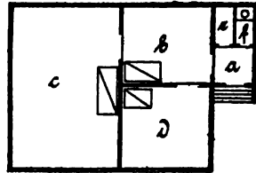
Fig. 3. Einfamilienhaus. a Vorraum. — b Küche. — c Stube. — d Kammer. — e Besenraum. — f Kloset.
