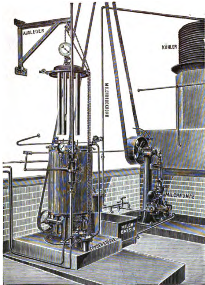
Fig. 1. Pasteurisir-Apparat.
