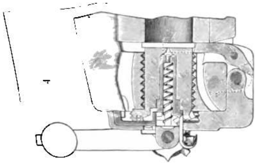
3 u. 4. Schraubenschluß für Schnellfeuergeschütze nach Maxim-Nordenfeli.
