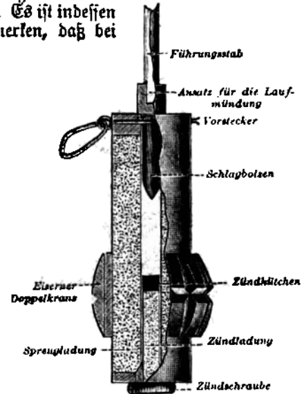
Fig. 4. Gewehrgranate von Marten Hale.
