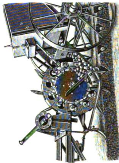
7. Kartoffellegemaschine von Gebr. Lesser, Posen.
