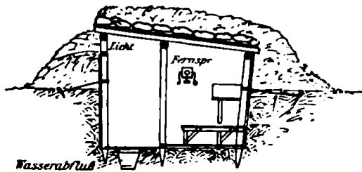
9 und 10. Fernsprechunterstand.
