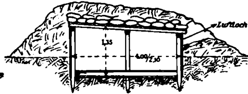
4. Schlafunterstand.
