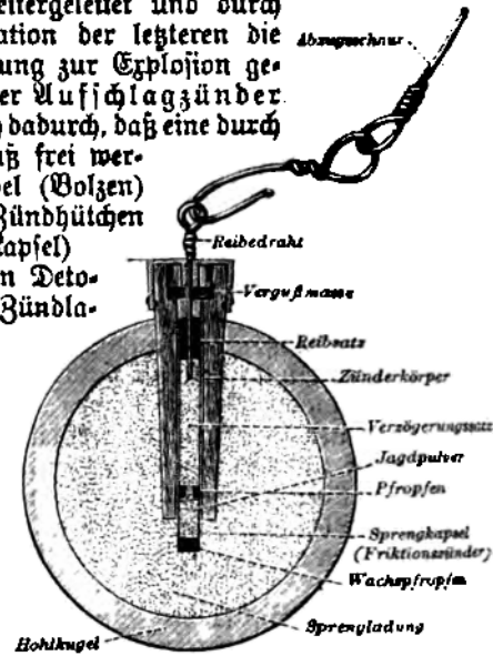
Fig. 1. Französische Handgranate mit Zeitzündung.
