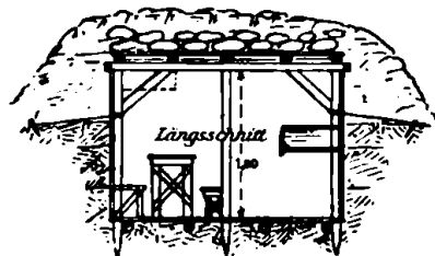
7 und 8. Unterstand für den Kompanieführer.
