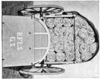
2. Gerätewagen 1895 des Feldlazarets, Packung nach Beinhelien.
