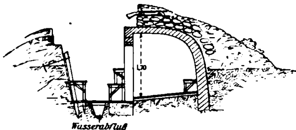
13 und 14. Eisenbetonunterstand.
