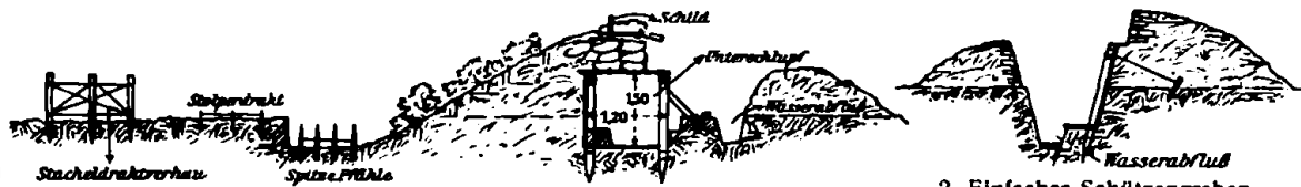
1. Vollständige Schützengrabenanlage mit Unterstand.
