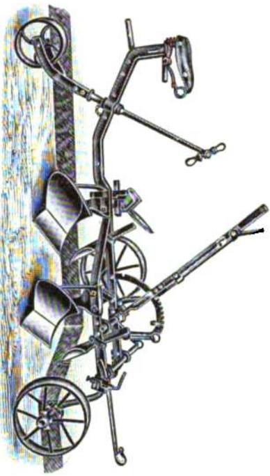
1. Zweischariger Sitzpflug der oberbayer. Pflugfabrik in Landsberg.
