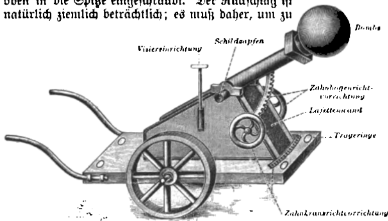
Fig. 7. Minenwerfer.
