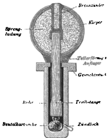
Fig. 8. Kugelförmige Bombe.
