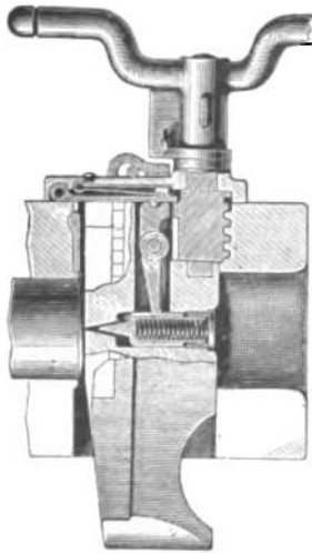
1. Krupp'scher Horizontalkeilverschluß für Schnellfeuerkanonen, in der Mitte wagrecht durchgeschnitten.
