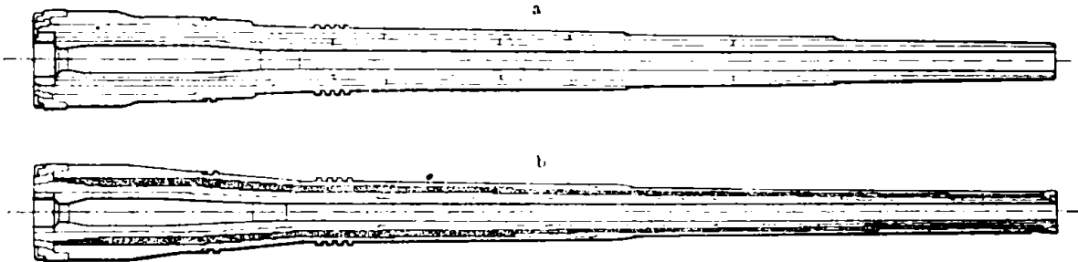
Fig. 1: a) 80,5 cm L/50 Mantelringrohr der Firma Biders; Rohrlänge 15,7 m. — b) 80,5 cm L/50 Drahtrohr der Firma Biders; Rohrlänge 15,7 m.
