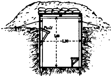
7 und 8. Unterstand für den Kompanieführer.
