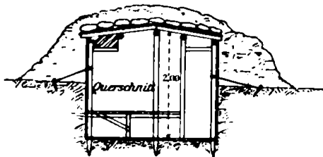
11 und 12. Verbandstelle.
