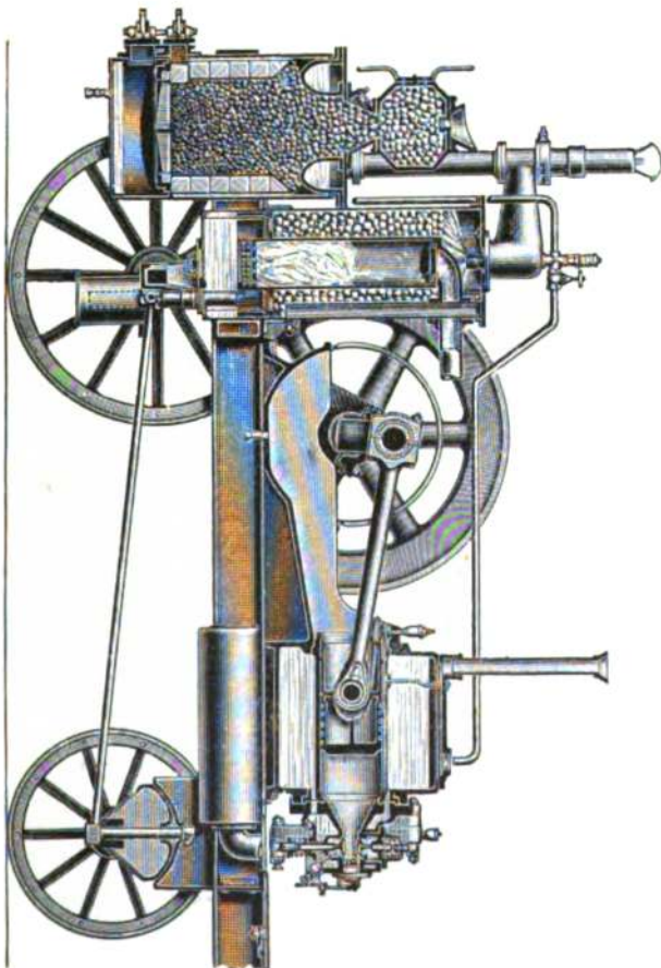
3. Sauggaslokomobile, Längsschnitt.
