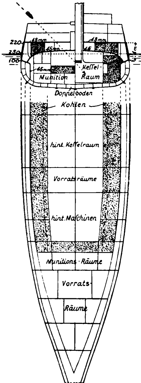
Fig. 4. Panzerschutz und Heißsystem eines franzö-sischen Linienschiffes.
